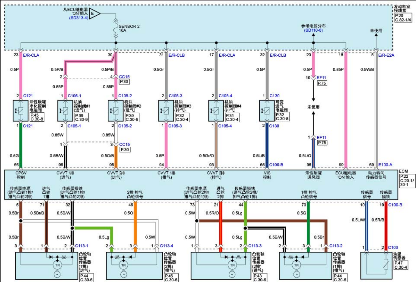
发动机控制系统(G6DJ : LAMBDA-II 3.8L GDI)(5)
